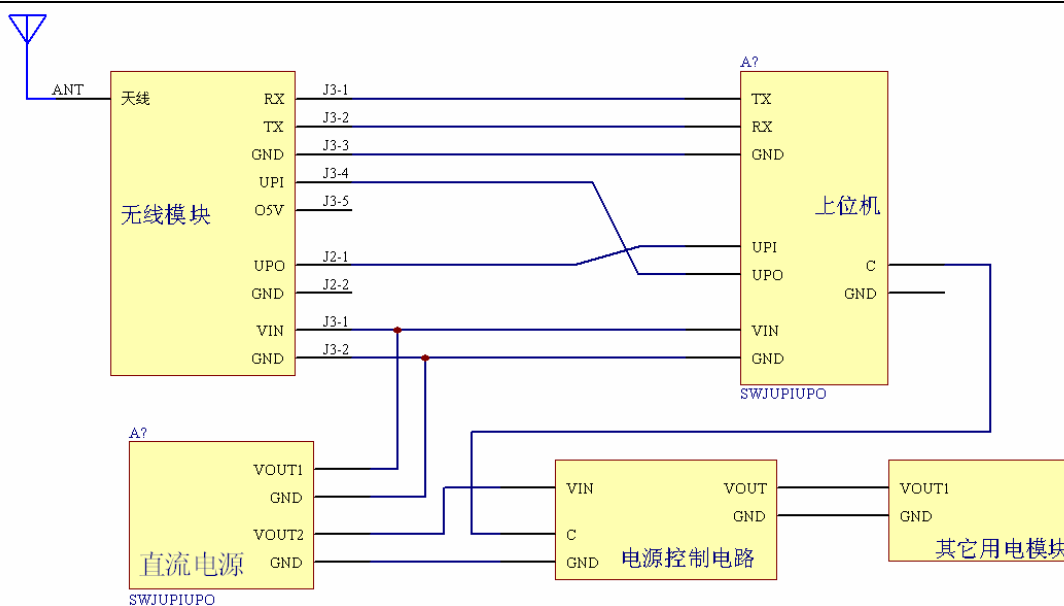
省电方式下空间唤醒控制电源电路的连接方法
